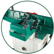
Guía escantillón ajustable de -45 a 45°.
